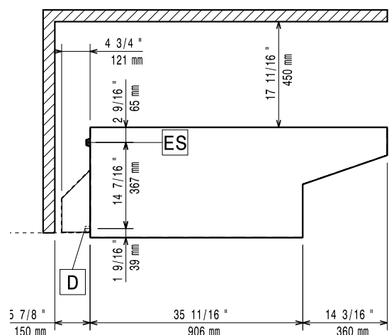
Bočna/o
